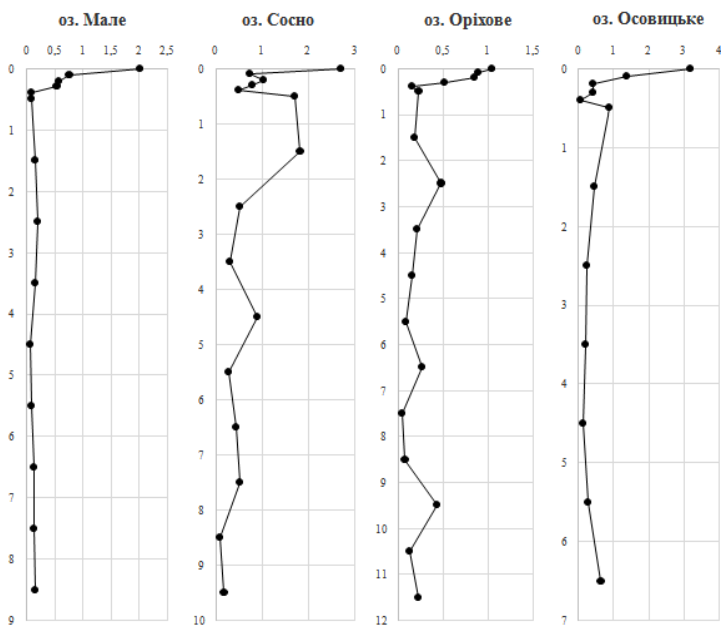
Рис. 1. Розподіл ^{137}\text{Cs} у донних відкладах озер, \text{Ki}/\text{kg} \cdot 10^{-9}
