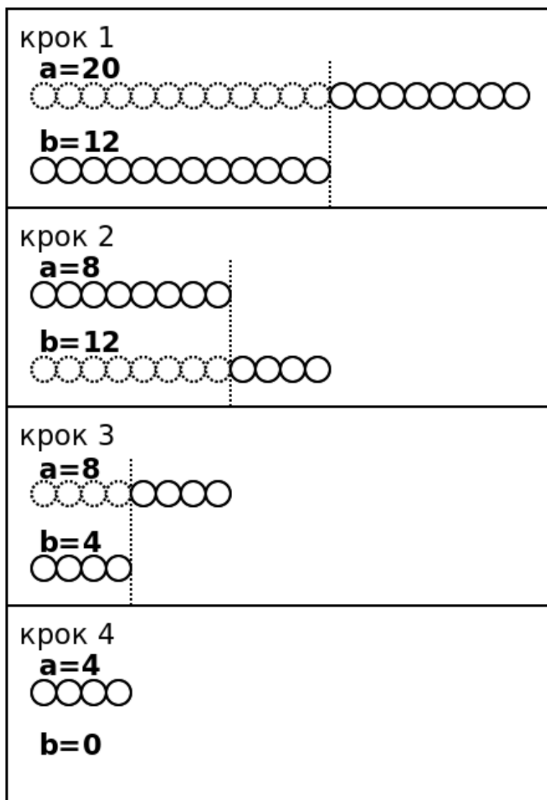
Схема виконання алгоритму пошуку НСД двох чисел
